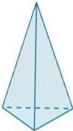
Pirámide triangular
