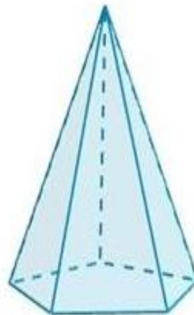
Pirámide pentagonal
