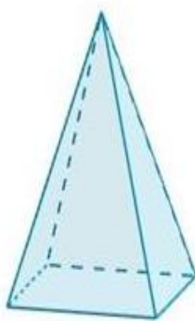
Pirámide cuadrangular
