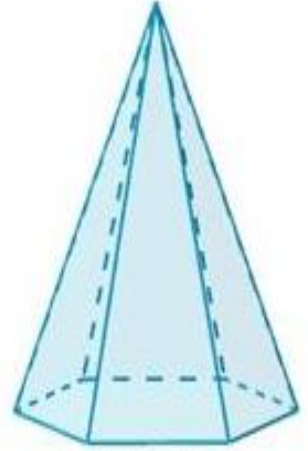
Pirámide hexagonal
