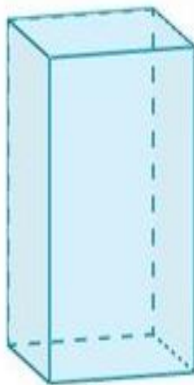
Prisma cuadrangular
